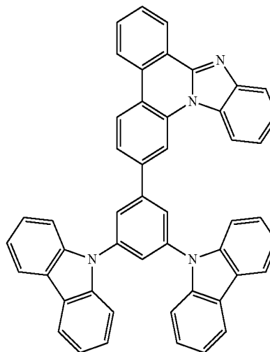
[GH]
